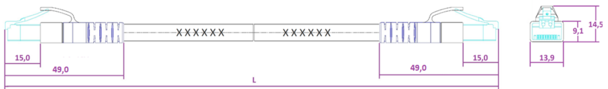
Maßzeichnung
