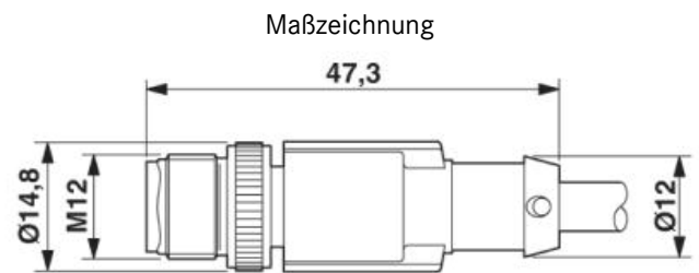
Stecker M12 x 1, gerade, geschirmt
