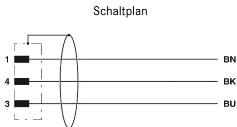
Kontaktbelegung des M12-Steckers
