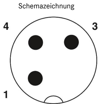
Polbild M12-Stecker, 3-polig, A-kodiert, Ansicht Stiftseite
