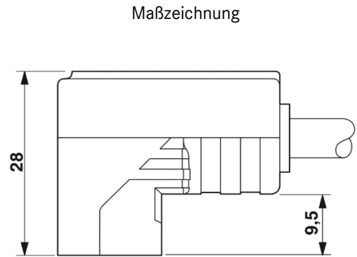
Ventilstecker, Bauform CI, Seitenansicht
