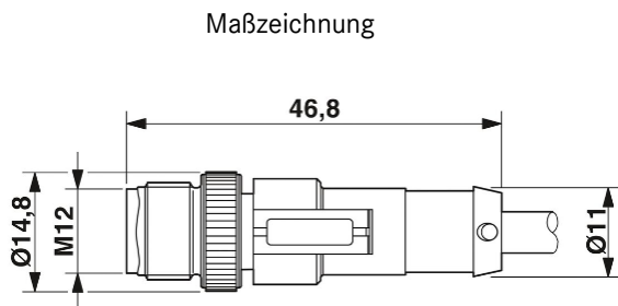
Stecker M12 x 1, gerade, A-kodiert
