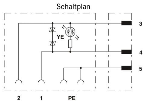
Kontaktbelegung des M12-Steckers und des Ventilsteckers
