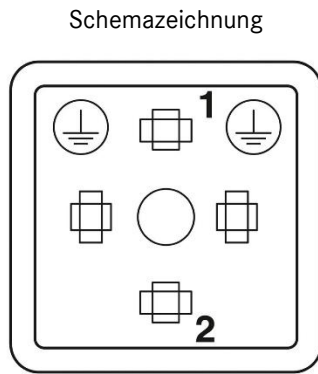
Polbild Ventilstecker, Bauform CI
