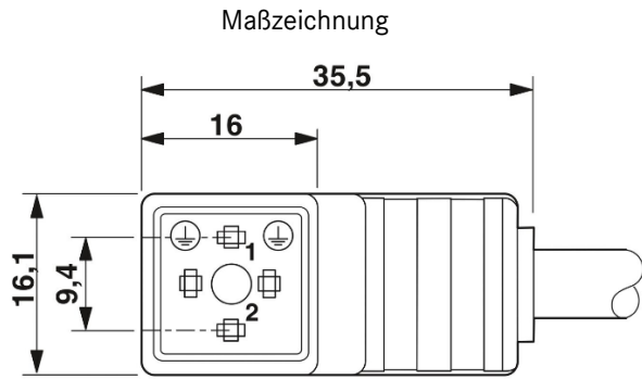
Ventilstecker, Bauform CI
