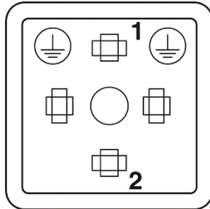
Polbild Ventilstecker, Bauform CI
