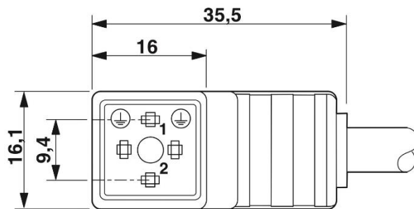
Ventilstecker, Bauform CI
